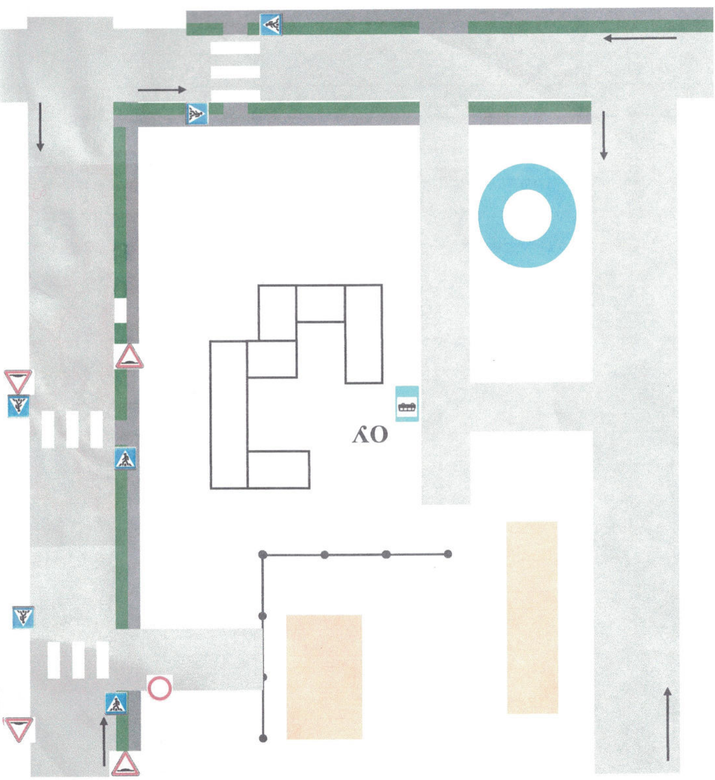
2. Схема организации дорожного движения в непосредственной близости от ОУ с размещением соответствующих технических средств организации дорожного движения, маршрутов движения детей
